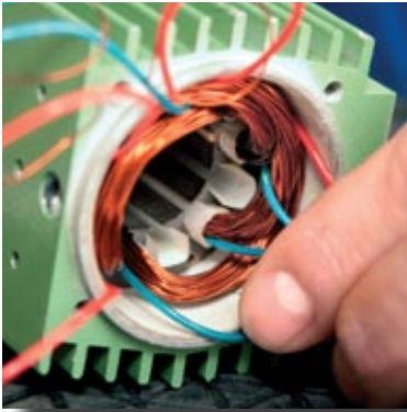
Miniwicklung Perske-Motor
